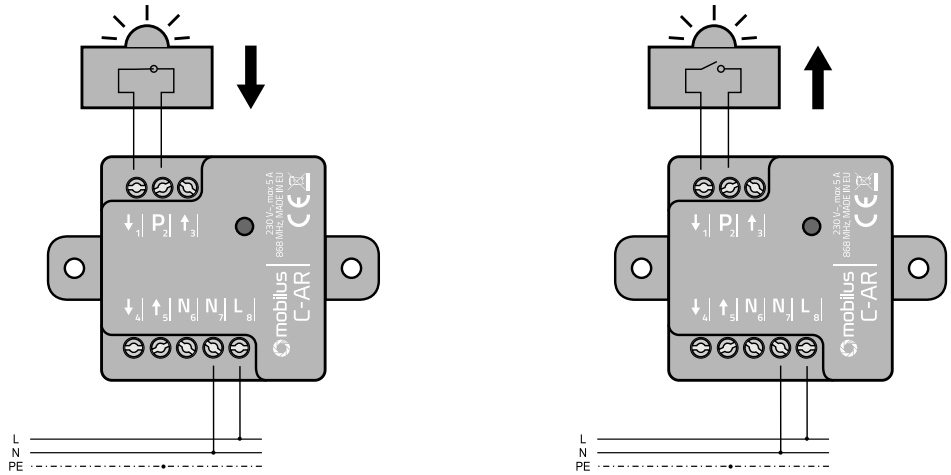
CIĄGŁY TRYB PRACY. Zwarcie wejścia 1 i 2 - wysyłanie rozkazu DÓŁ. CIĄGŁY TRYB PRACY. Rozwarcie wejścia 1 i 2 - wysyłanie rozkazu GÓRA
